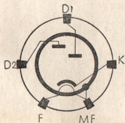
Sockelschaltung
