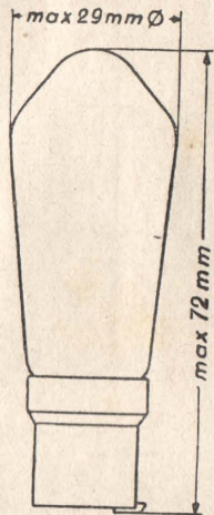
Kolbengrösse
